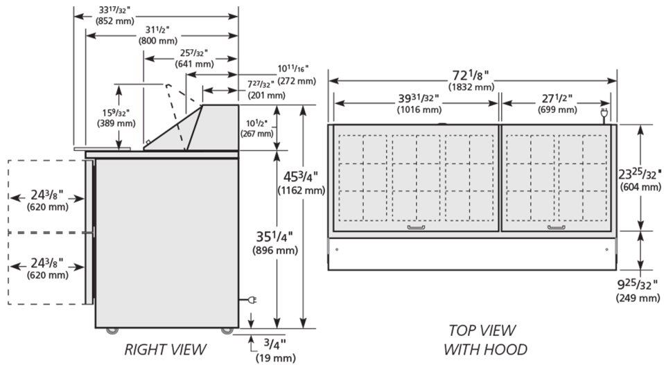
ELEVATION
